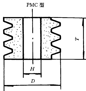
图 1 砂轮剖面图
